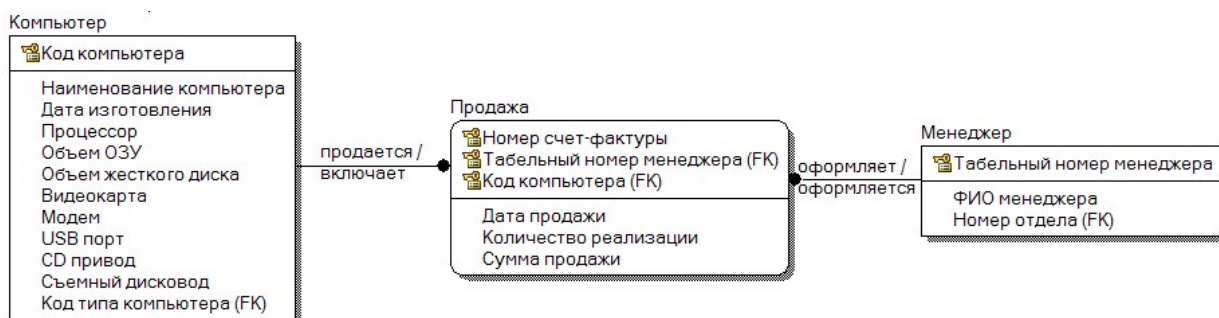
Рисунок 2. Связь между сущностями Компьютер, Продажа и Менеджер
