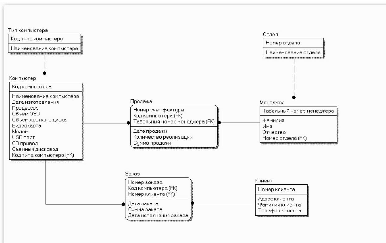
Рисунок 4. Логическая модель данных системы «Реализация средств вычислительной техники»
